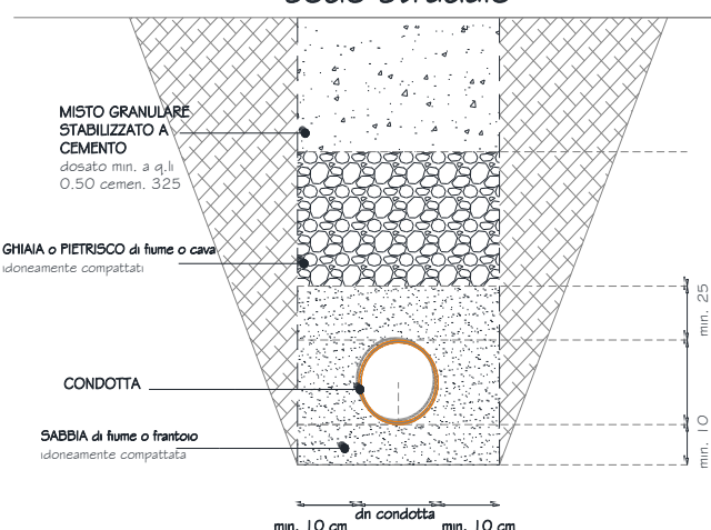
sezione tipo su sede stradale
